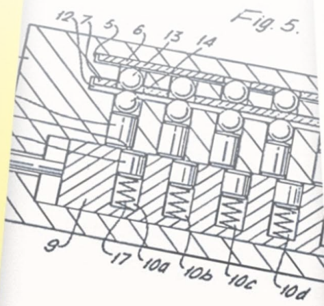
Den første prototypen på VingCard låsen.
